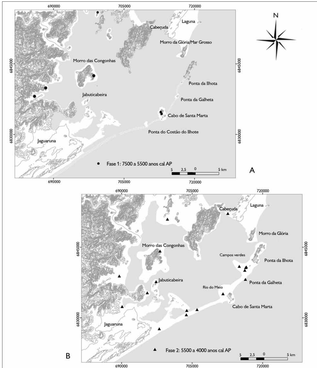
Figura 6. Mapas de distribuição de sambaquis contendo material datado em fases anteriores a 4.000 anos AP: A) Fase 1: intervalo entre 7.500 e 5.500 anos cal AP; B) Fase 2: intervalo entre 5.500 e 4.000 anos AP. A barreira transgressiva inicial deve ter-se formado no decorrer da fase 1, numa posição possivelmente mais ao mar que a atual.
